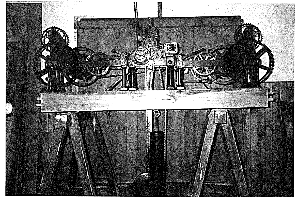
Mécanisme de l'ancienne horloge.
