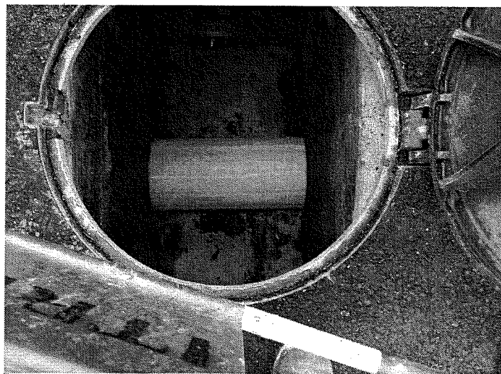
Perçage des raccords avec un robot Passage de la caméra pour contrôle Mise en place d'un manchon sur chaque raccordement avec un robot.
